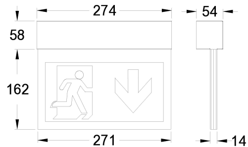
Maßzeichnung (Angaben in mm)
