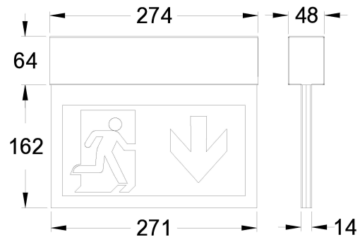
Maßzeichnung (Angaben in mm)
