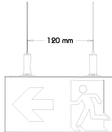
Ansicht Hinten
