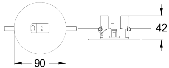
Maßzeichnung (Angaben in mm)
