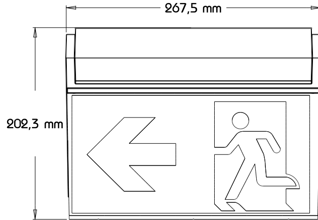
Ansicht Vorne
