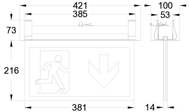
Maßzeichnung (Angaben in mm)
