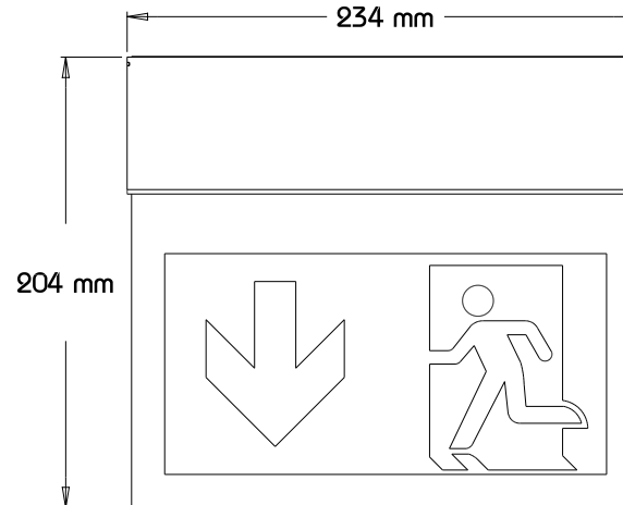
Ansicht Hinten
