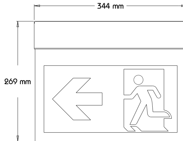
Ansicht Hinten
