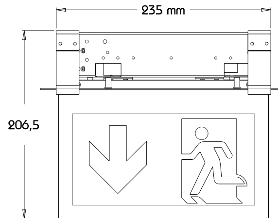
Ansicht Hinten
