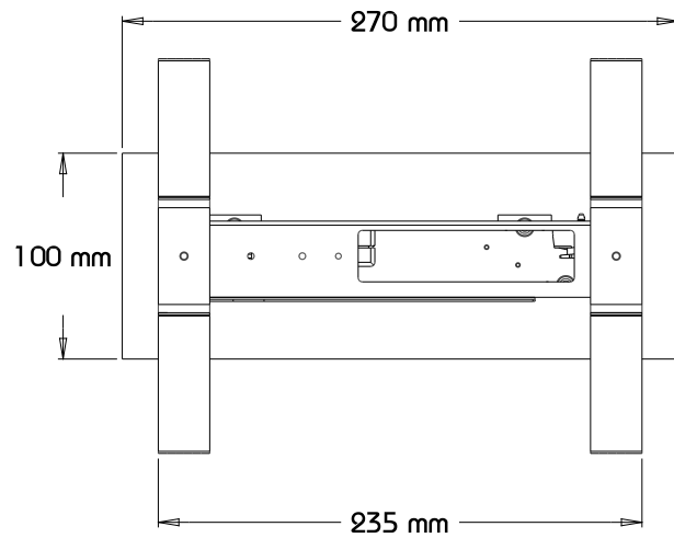
Ansicht Oben
