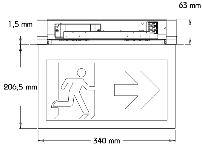
Ansicht Vorne
