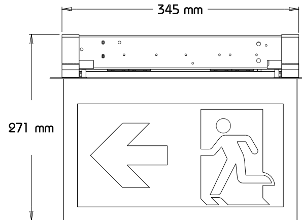
Ansicht Hinten
