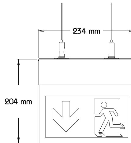
Ansicht Hinten
