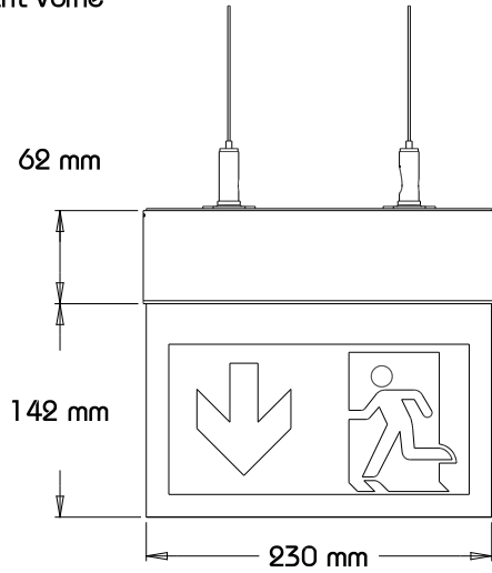
Ansicht Vorne
