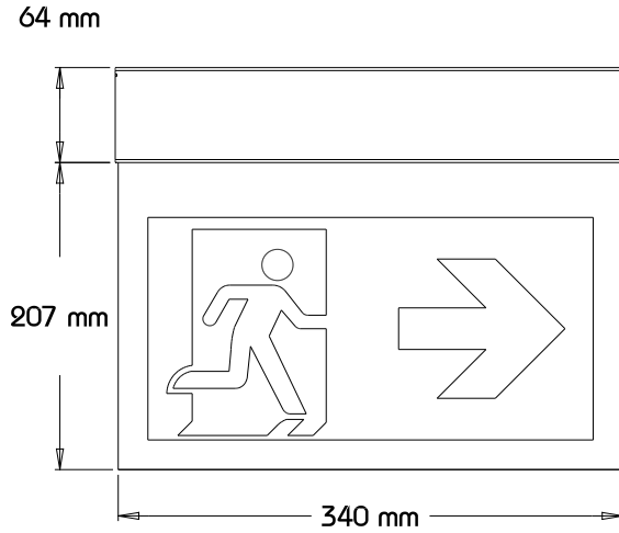
Ansicht Vorne
