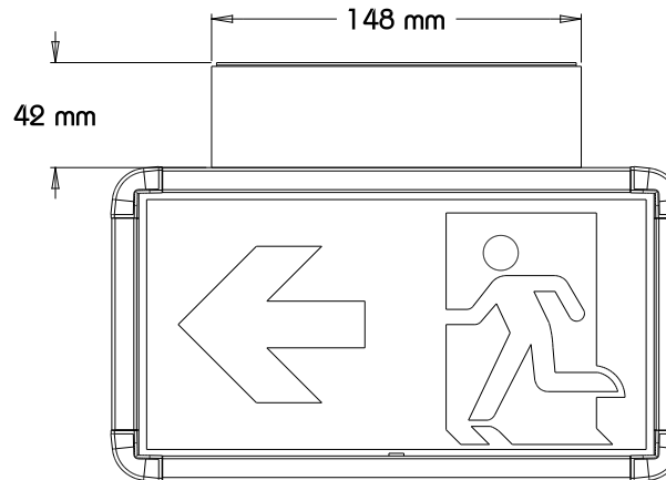
Ansicht Hinten
