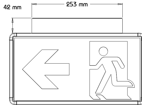
Ansicht Hinten
