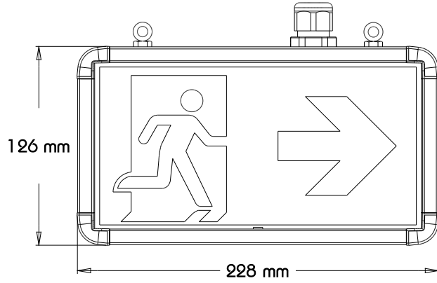
Ansicht Vorne
