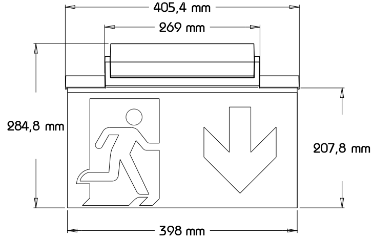
Ansicht Vorne
