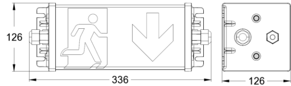
Maßzeichnung (Angaben in mm)
