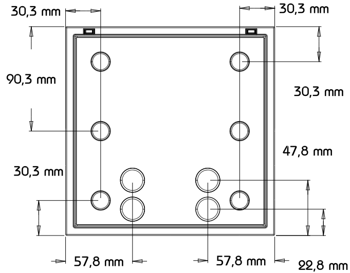
Ansicht Oben
