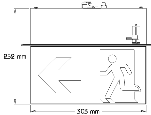
Ansicht Hinten
