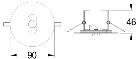
Maßzeichnung (Angaben in mm)
