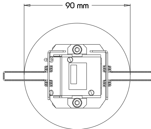
Ansicht Oben
