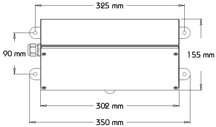
Ansicht Oben
