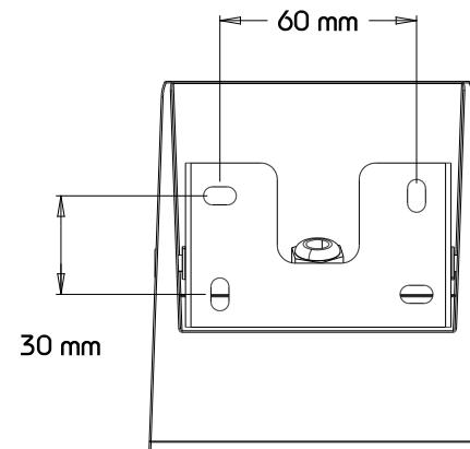
Ansicht Hinten
