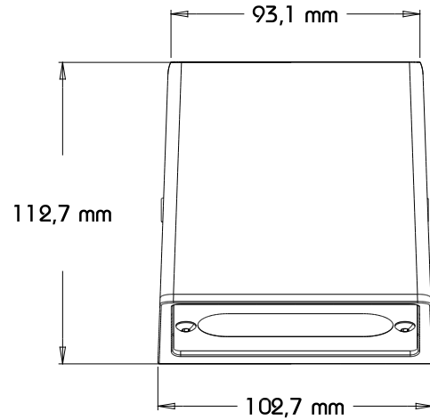
Ansicht Vorne
