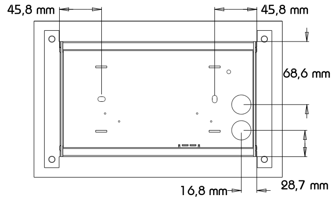
Ansicht Hinten
