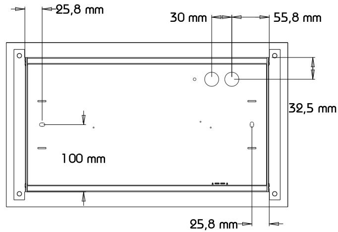
Ansicht Hinten
