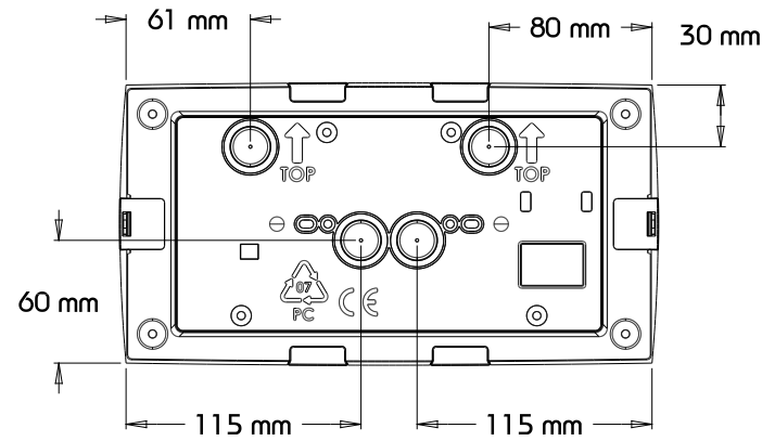
Ansicht Hinten
