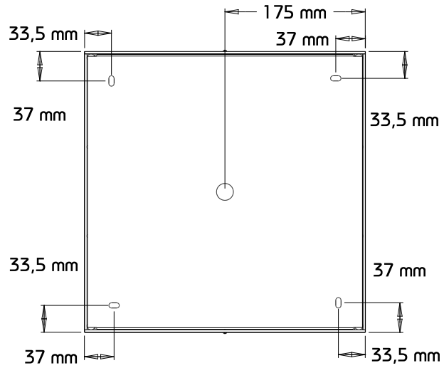
Ansicht Oben
