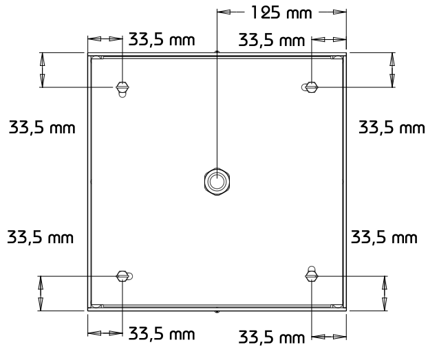
Ansicht Oben
