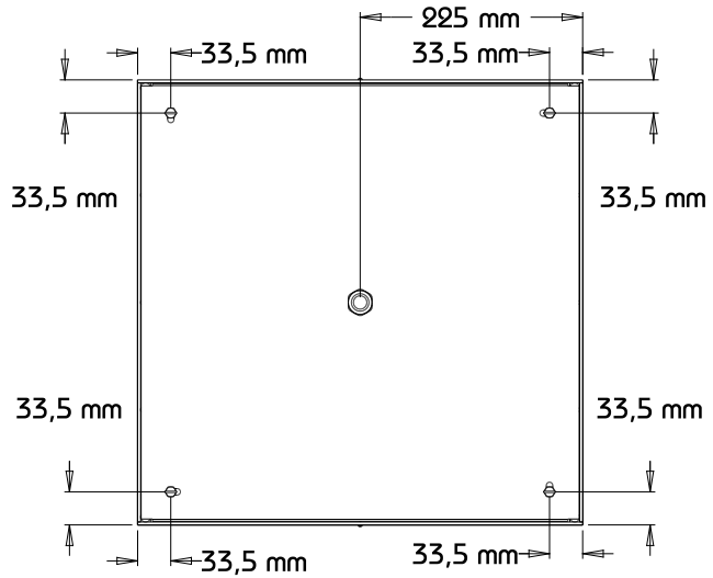
Ansicht Oben
