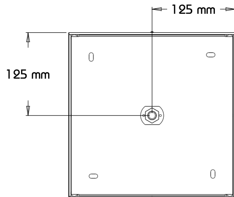
Ansicht Oben
