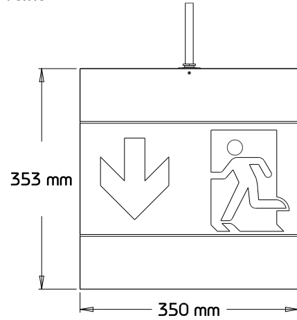
Ansicht Vorne
