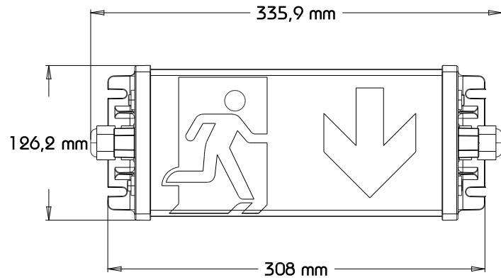
Ansicht Vorne
